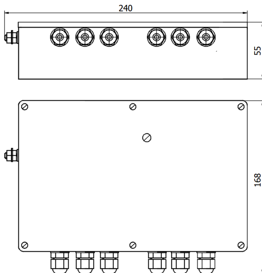
Рисунок 1 - Габаритный чертеж корпуса
